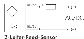
2-Leiter-Reed-Sensor
