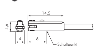
2-Leiter-Reed-Sensor
