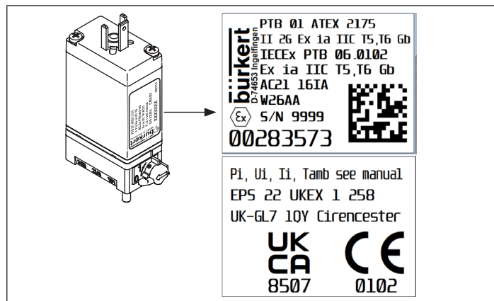
Bild 1: Lage und beispielhafte Darstellung des Typschilds
